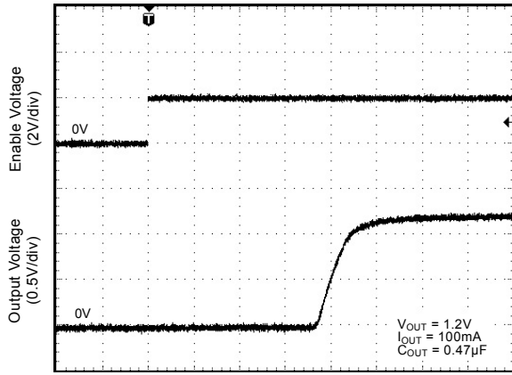
Enable Turn-On Transient
